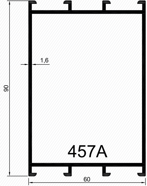
Geniş Kasa Profili - Frame Profile
