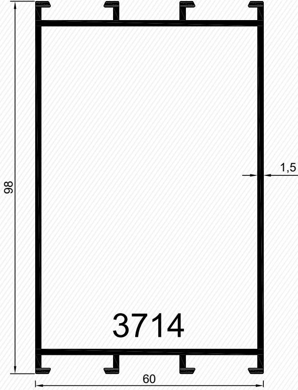
Köşe Dönüş Profili - Corner Profile
