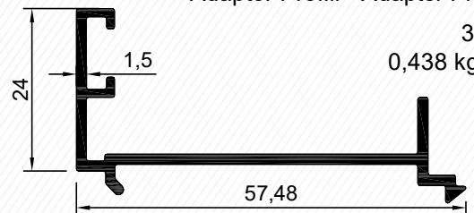
Adaptör Profili - Adapter Profile
