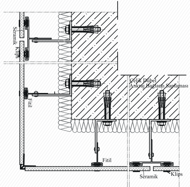
Dış Köşe Detayı
