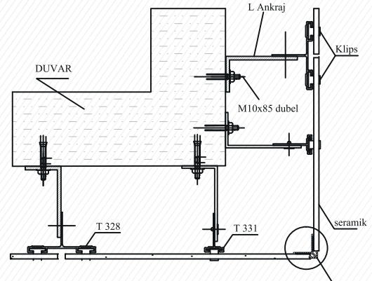
Dış Köşe Detayı
