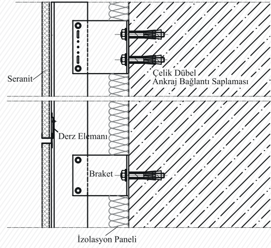
Düşey Kesit
