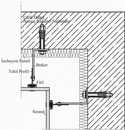
İç Köşe Detayı
