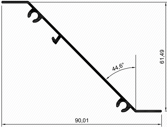
506 0,496 kg/m
