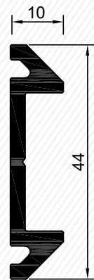
3448 0,495 kg/m
