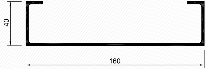
3951 1,777 kg/m
