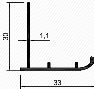
3231 0,213 kg/m
