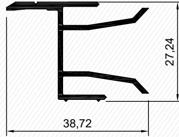
3378 0,387 kg/m
