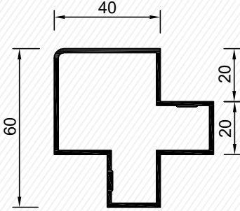
3949 0,967 kg/m
