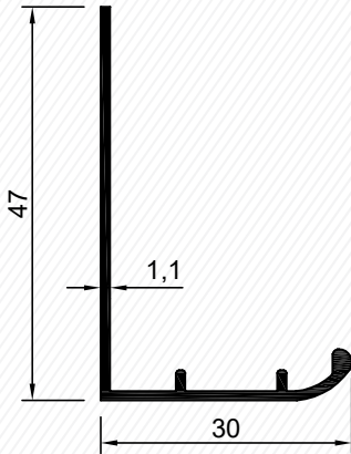
3230 0,233 kg/m
