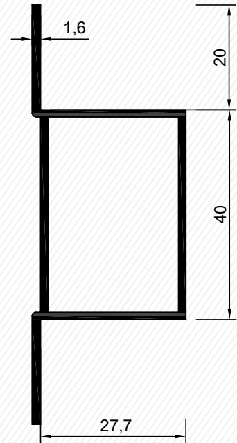
3317 0,678 kg/m
