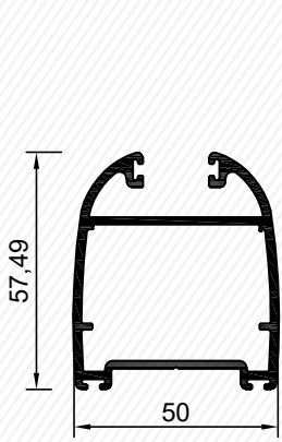
3449 1,305 kg/m
