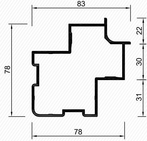
3948 1,6342 kg/m
