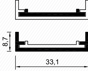
3356 0,107 kg/m
