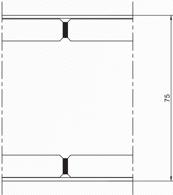
2 mm VHB Bant ile - Cam Camu Birleşim Detayı 2 mm with VHB Band - Glass & Glass Assembly Detail
