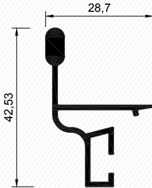
Sineklik Çıta Profili - Fly Screen Beat Profile
