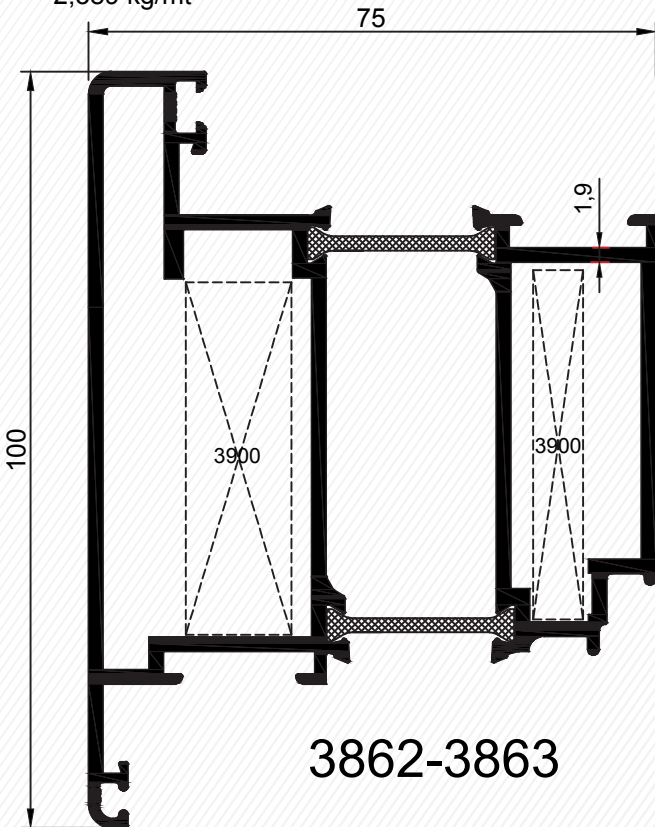
Dışa Açılım Kapı Kanat - Door Sash Profile
