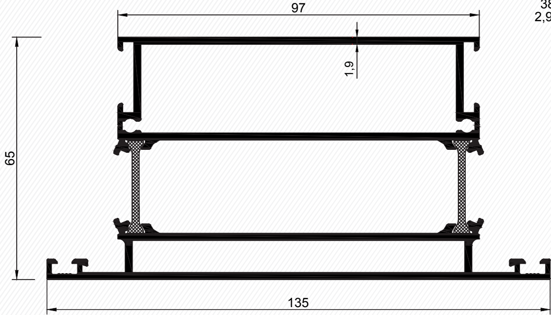
Duple Orta Kayıt Profili - Double Mullion Profile
