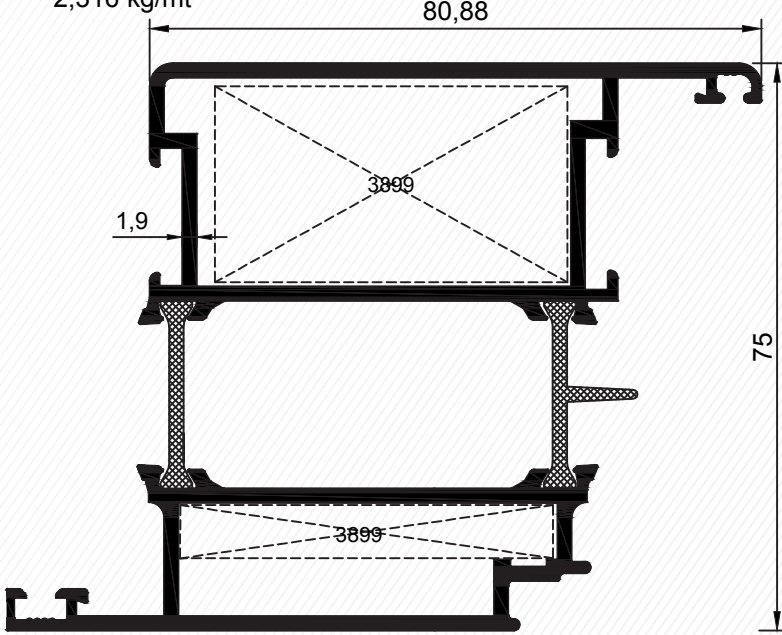
Kapı Kanat Profili - Door Sash Profile
