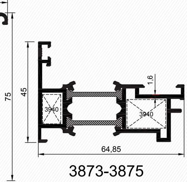
Dışa Açılım Adaptör Profili - Adapter Profile
