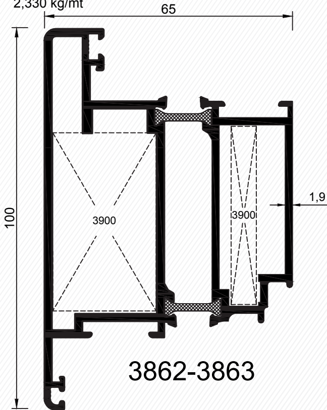
Dışa Açılım Kapı Kanat Profili - Door Sash Profile 3862-3863 2,330 kg/mt
