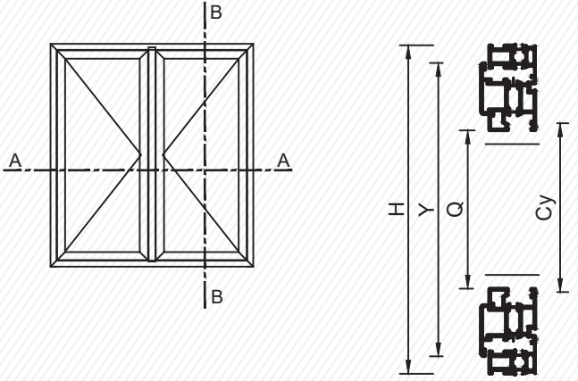
B-B KESİTİ / SECTION
