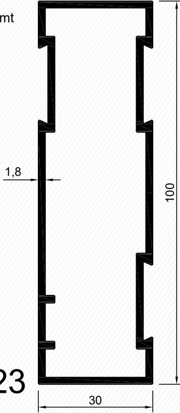
Kasa Profili - Frame Profile
