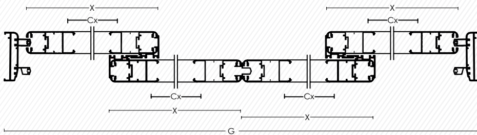
A-A KESİTİ / SECTION
