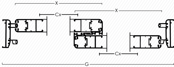
A-A KESİTİ / SECTION
