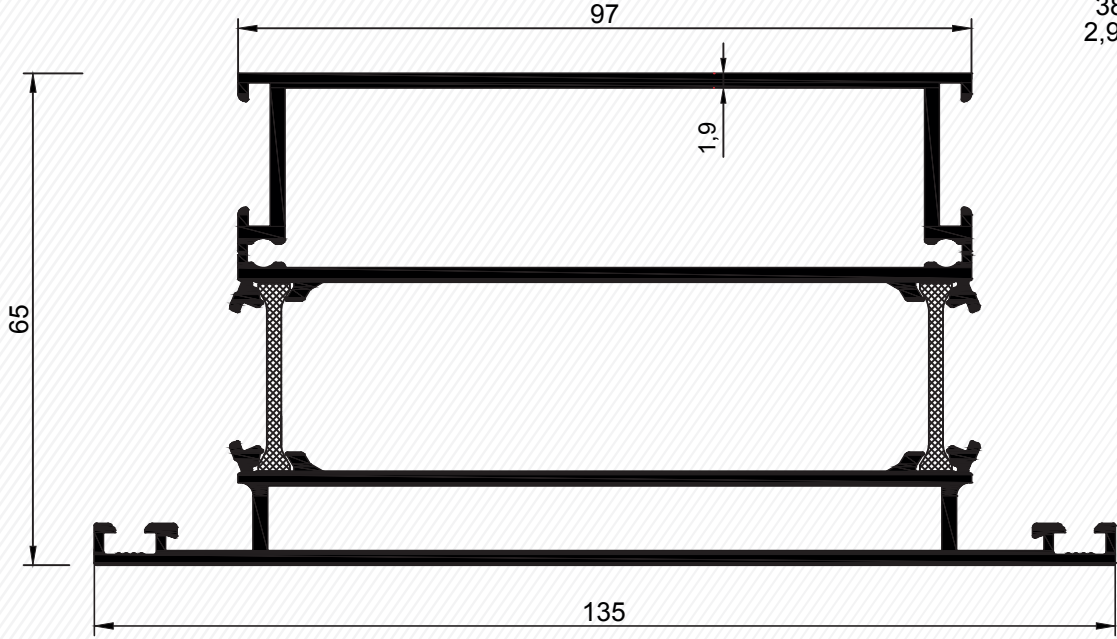
Duble Orta Kayıt Profili - Double Mullion Profile
