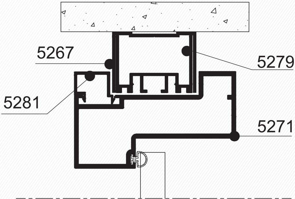
Kapı Kasası - Üst Detayı Door Frame- Head Detail
