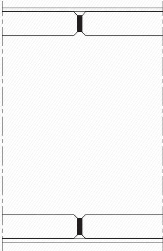
2 mm VHB Bant ile - Cam Cama Birleşim Detayı 2 mm with VHB Band - Glass & Glass Assembly Detail
