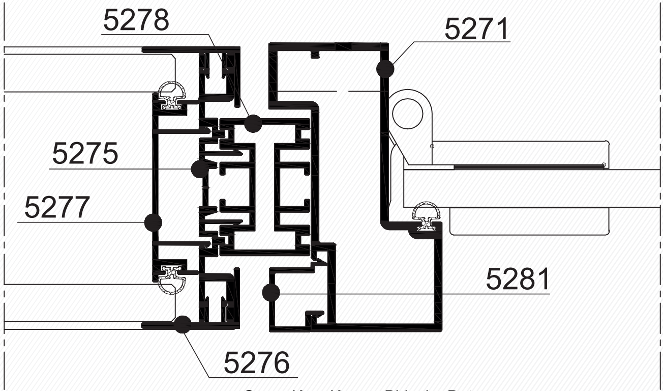
Cam - Kapı Kasası Birleşim Detayı Glass - Door Frame Assembly Detail
