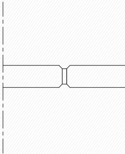
2 mm VHB Bant ile - Cam Cam Birleşim Detayı 2 mm with VHB Band - Glass & Glass Assembly Detail
