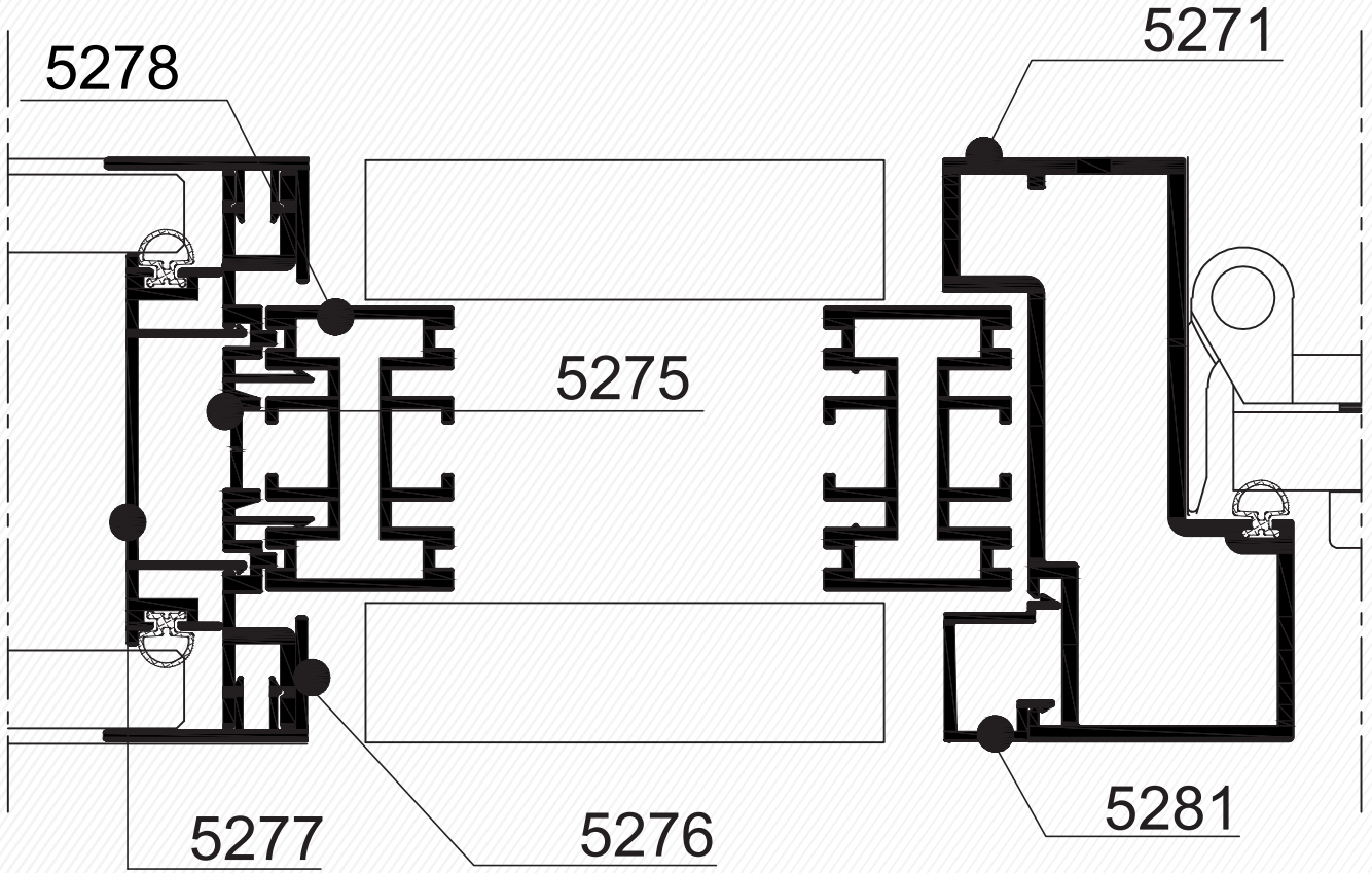
Kapı Kasası - Teknik Panel - Cam Birleşim Tetayı Door Frame - Technical Panel - Glass Assembly Detail
