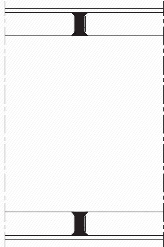
H Profil ile Cam Cama Birleşim Detayı With H Profile - Glass&Glass Assembly Detail
