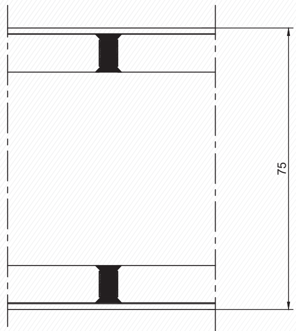
H Profil ile Cam Cam Birleşim Detayı With H Profile - Glass&Glass Assembly Detail
