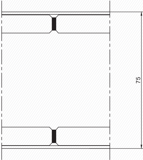
2 mm VHB Bant ile - Cam Cam Birleşim Detayı 2 mm with VHB Band - Glass & Glass Assembly Detail
