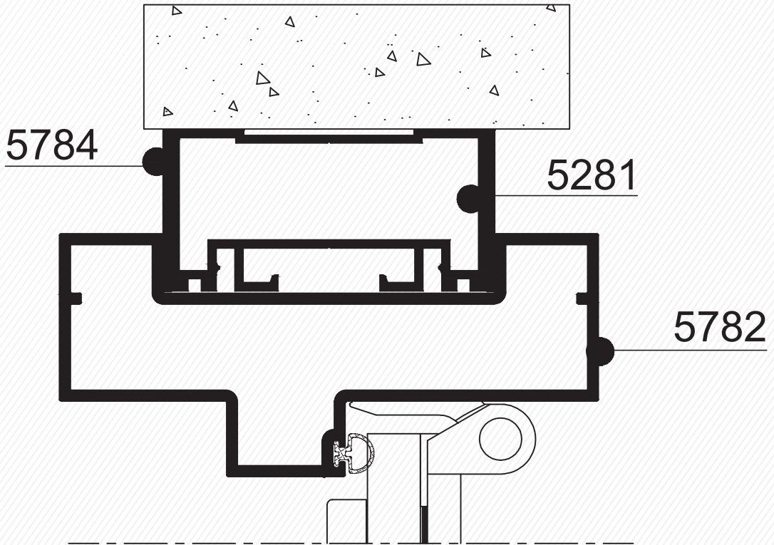
Kapı Kasası - Üst Detayı Door Frame- Head Detail
