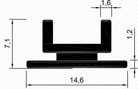
2348 0,131 kg/m
