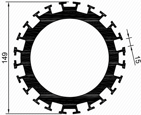
2346 14,491 kg/m
