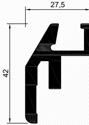
1984 0,957 kg/m
