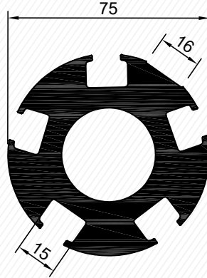
2347 6,895 kg/m
