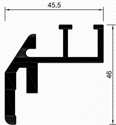
1985 0,198 kg/m
