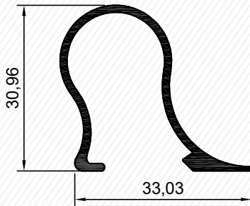
Tutamak Profili Handle Profile
