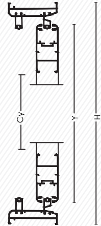
B-B KESİTİ / SECTION
