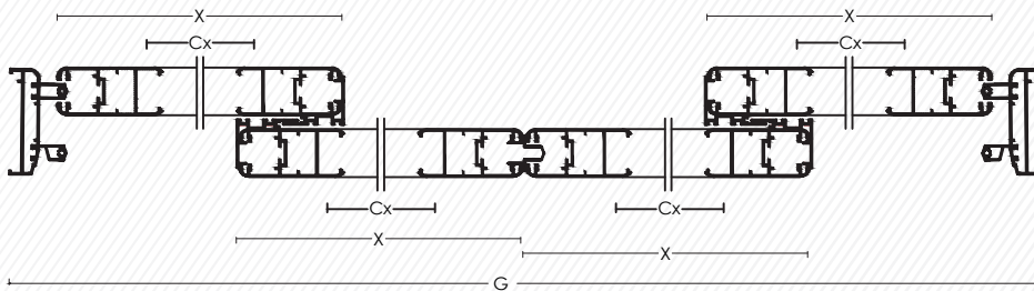
A-A KESİTİ / SECTION
