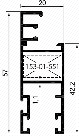
Sineklik Kanat Profili Fly Screen Sash Profile
