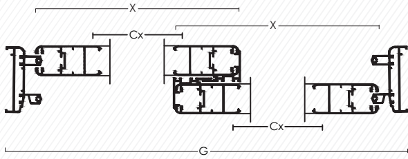
A-A KESİTİ / SECTION
