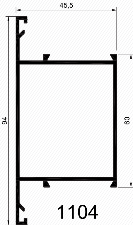
Orta Kayıt Profili - Middle Transom Profile
